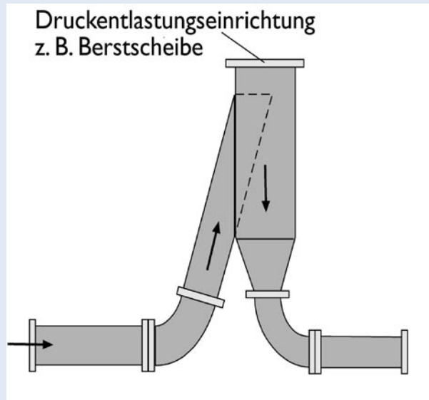
Bild 1: Schematische Darstellung eines Entlastungsschlotes
